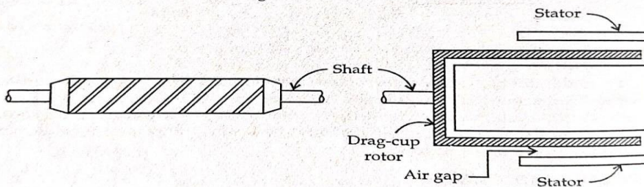
Fig. 9.4. a.c. servomotor
