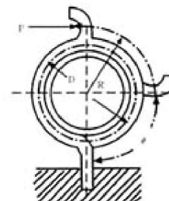
Torsion
